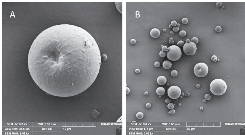
Obř. 7. Fotografie z elektronového mikroskopu PLGA mikročářtice z Resomeru ® 653 H; A) mikročářtice (měřítko 10 \mu\text{m} ), B) mikročářtice (měřítko 50 \mu\text{m} ) (Foto: J. Vysloužil).
